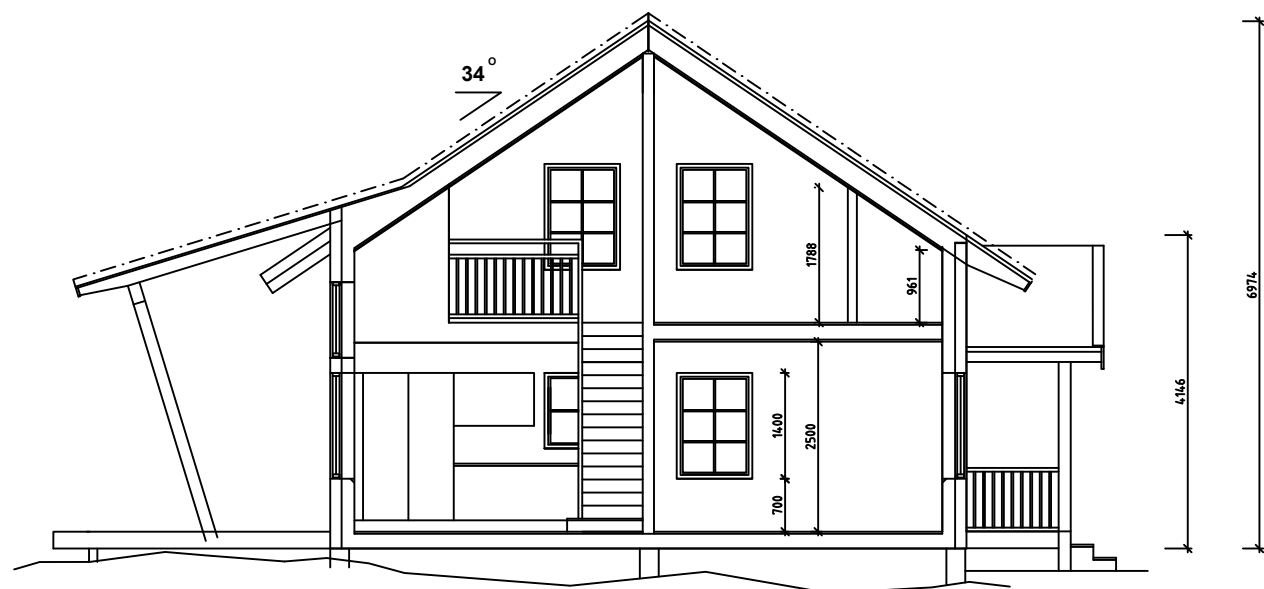
SEKTION A-A
