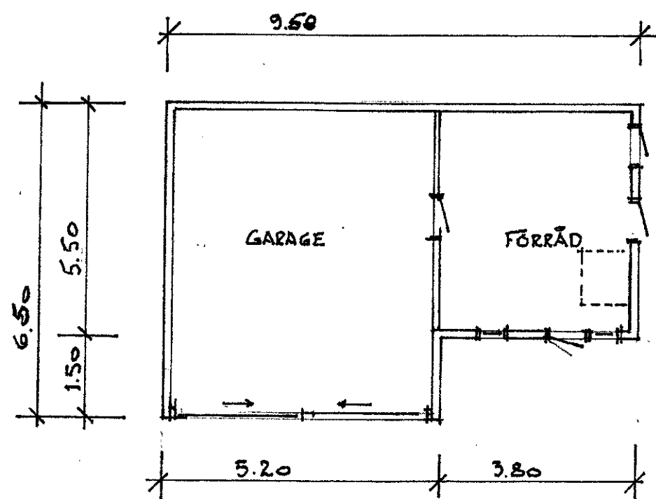
PLAN SK. 1:100
