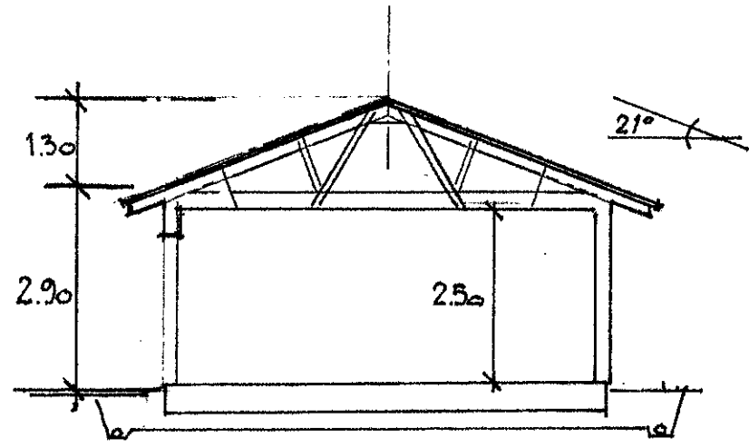
SEKTION SK. 1:100
