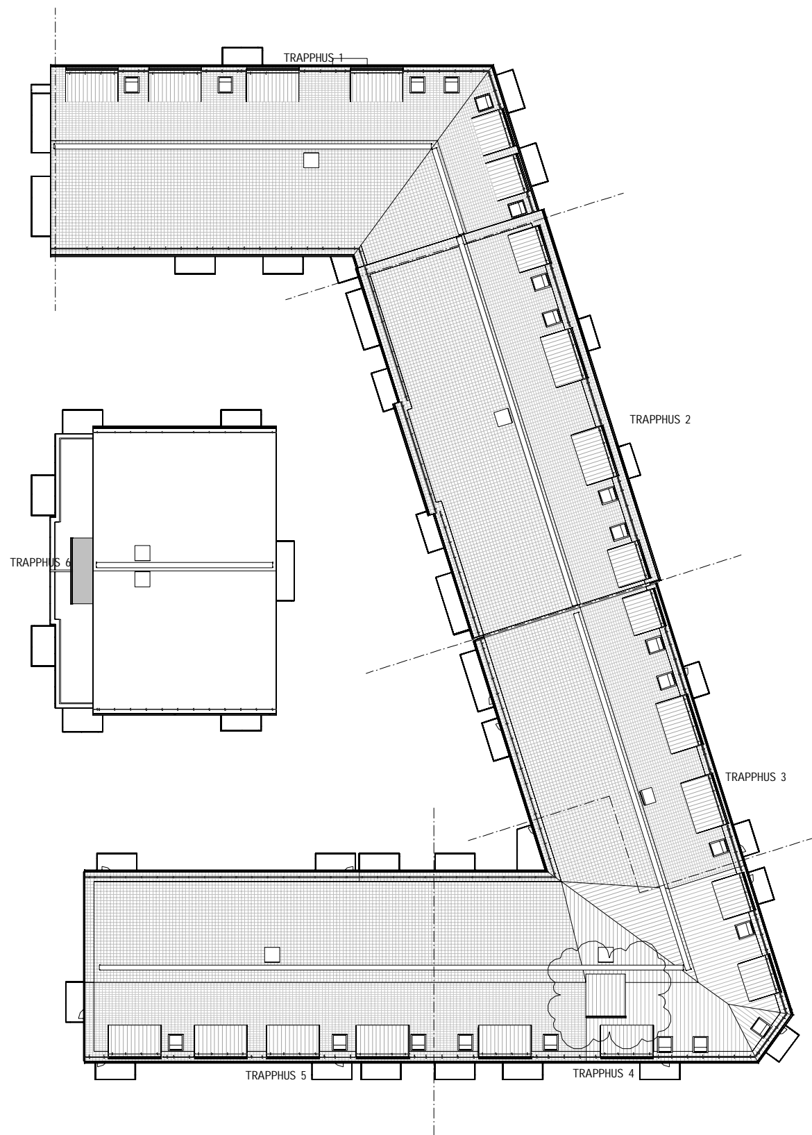
ÖVERSIKT TAKPLAN BL 1 : 200
