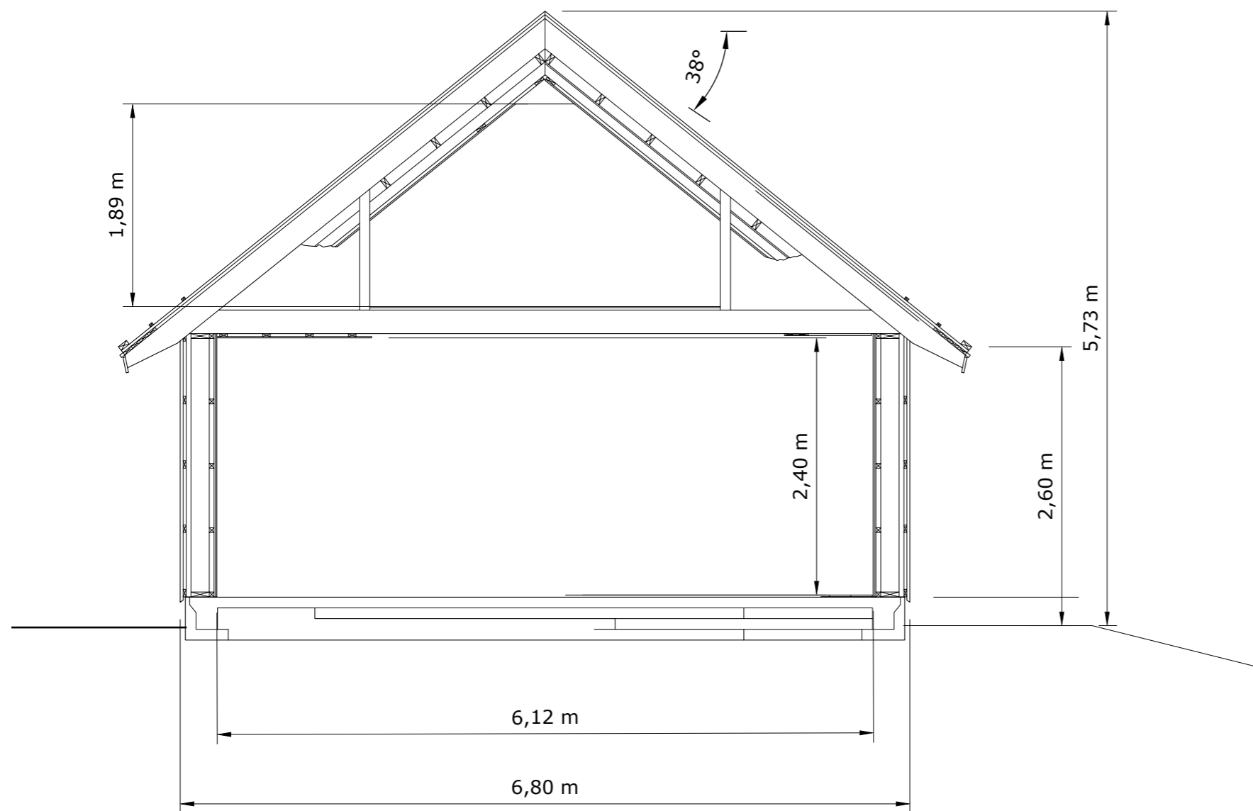
SEKTION A-A
