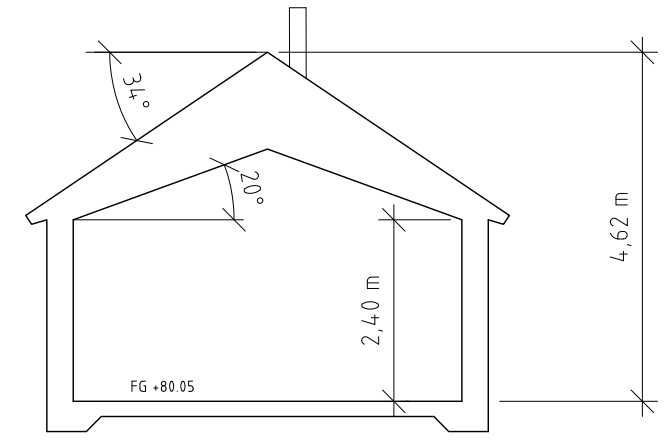
Sektion A-A
