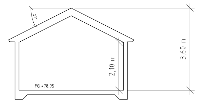
Sektion B-B
