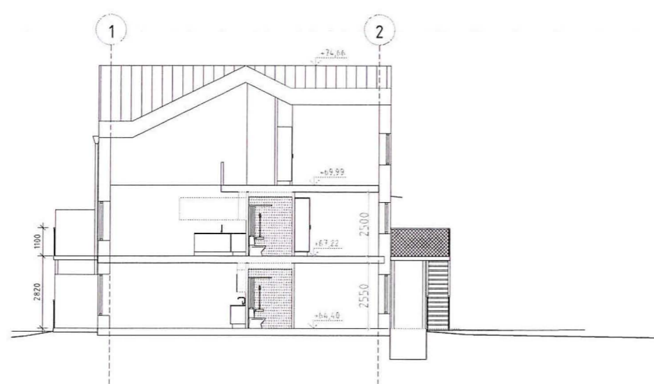
SEKTION B-B
