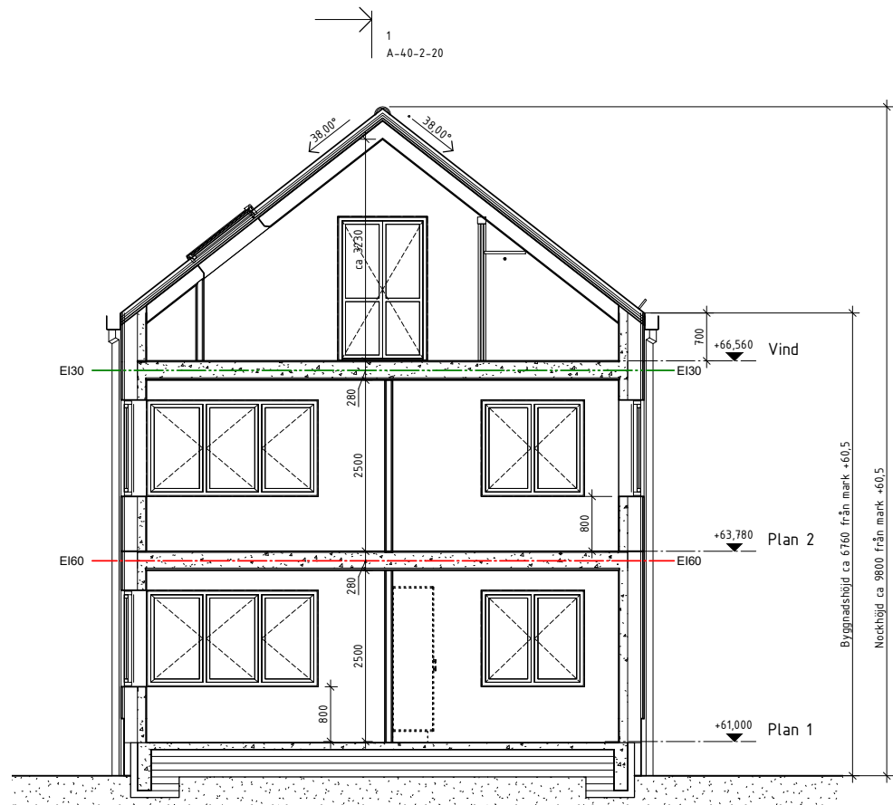
Tvärsektion A1
