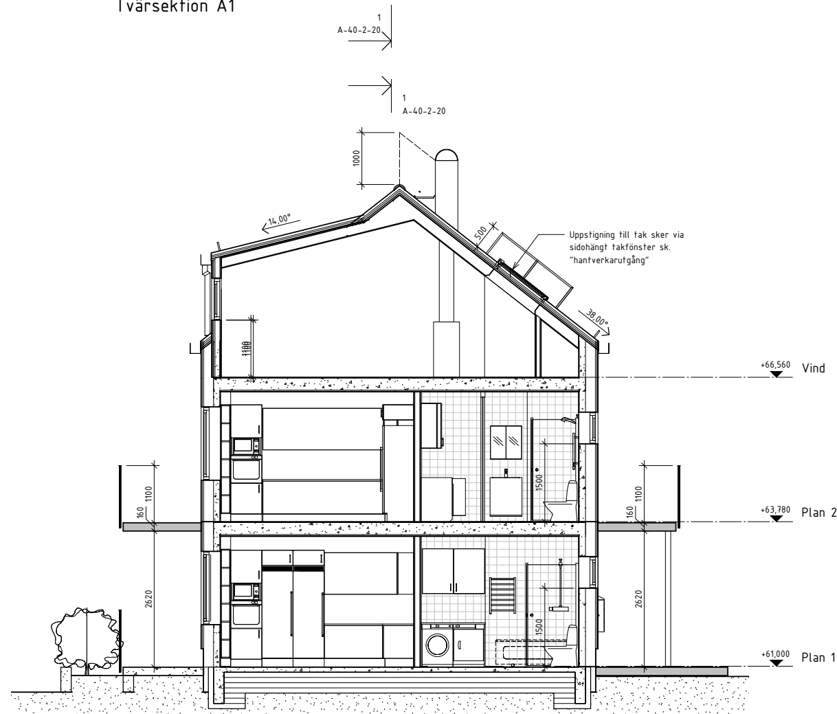
Tvärsektion A3
