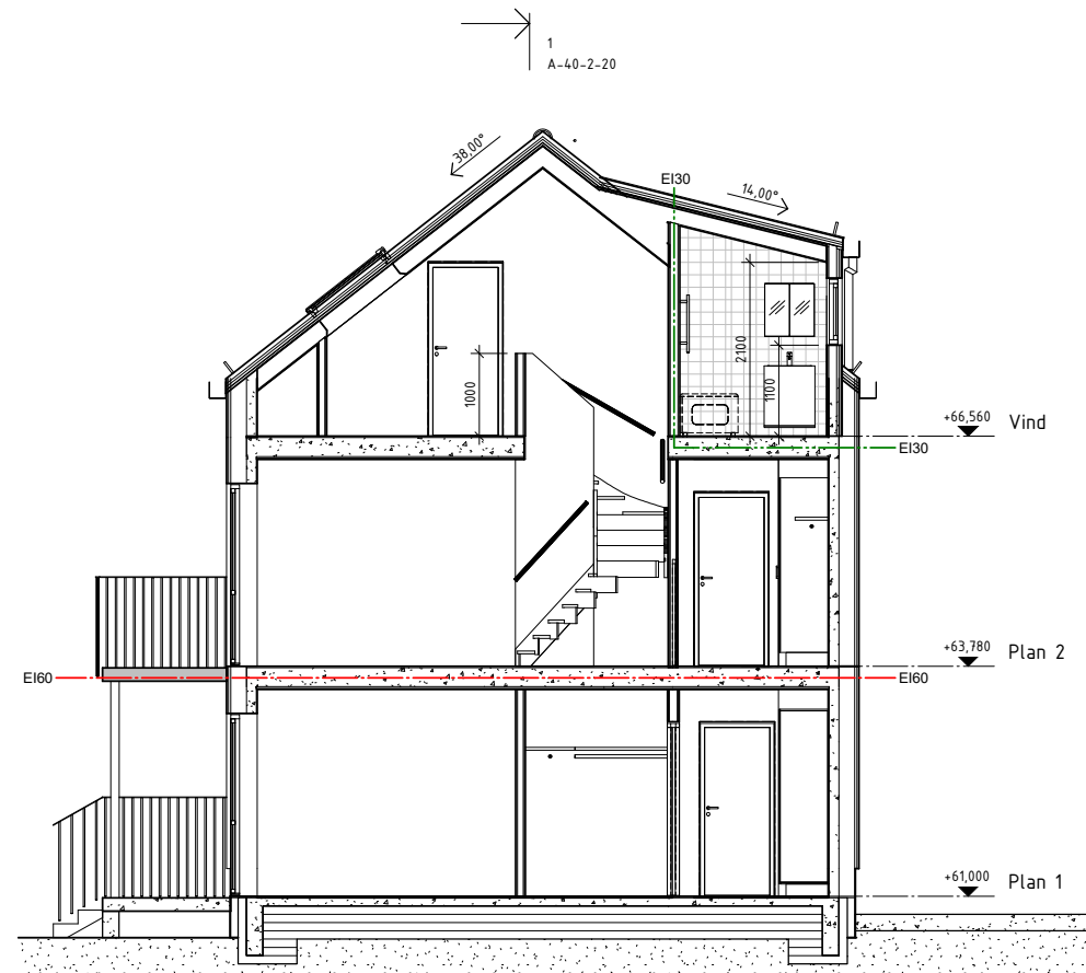
Tvärsektion A2
