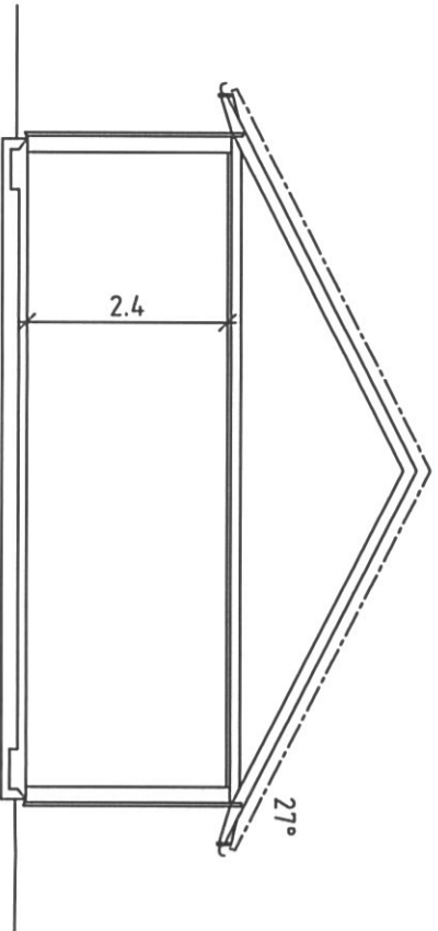
SEKTION
