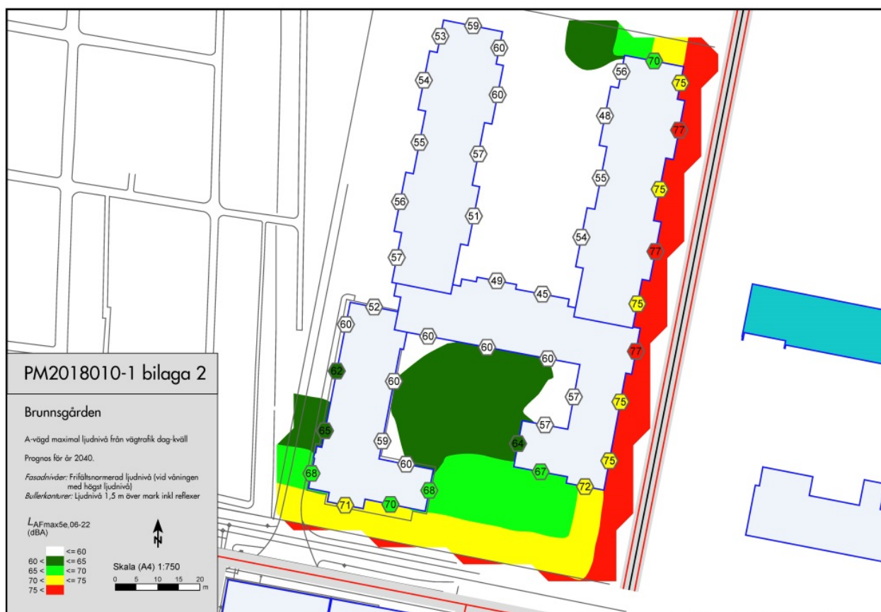
Gärdhagen Akustik 2018. A-vägd maximal ljudnivå från vägtrafik dag-kväll, prognos 2040.
