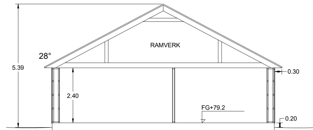
SEKTION A-A
