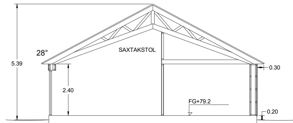
SEKTION C-C
