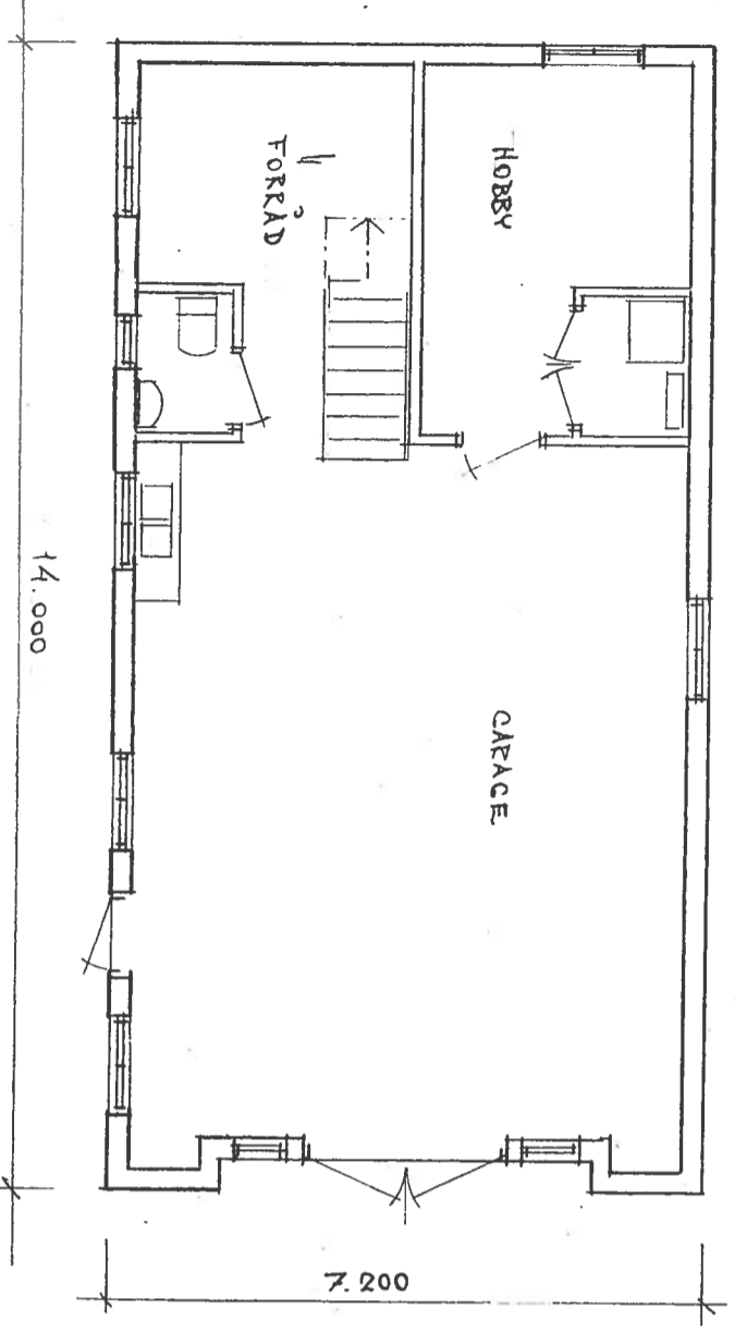
PLAN 1:100
