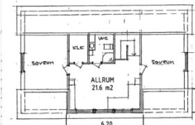
PLAN ÖVERVÅNING NYTILLKOMMEN BTA: 10,5 m² NYTILLKOMMEN ÖPPENARE: 10,5 m²
