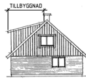
FASAD MOT NÖRÖST
