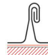
PRINCIPDETALJ DUBBEL STÅNDFALS
