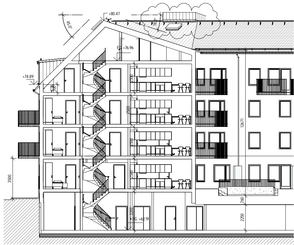
SEKTION C-C BL 1 : 100
