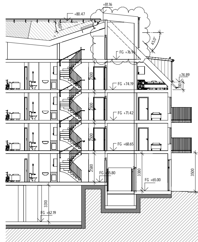
SEKTION D-D BL 1 : 100
