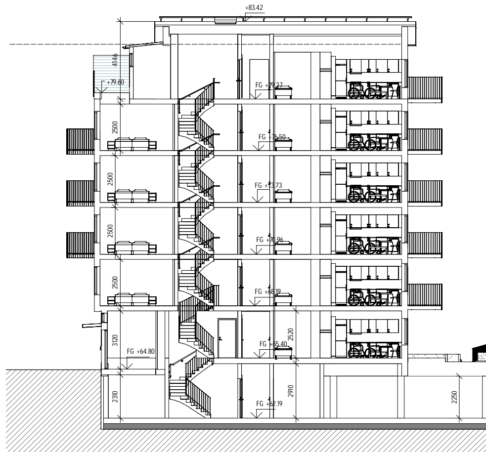
SEKTION C-C BL 1 : 100
