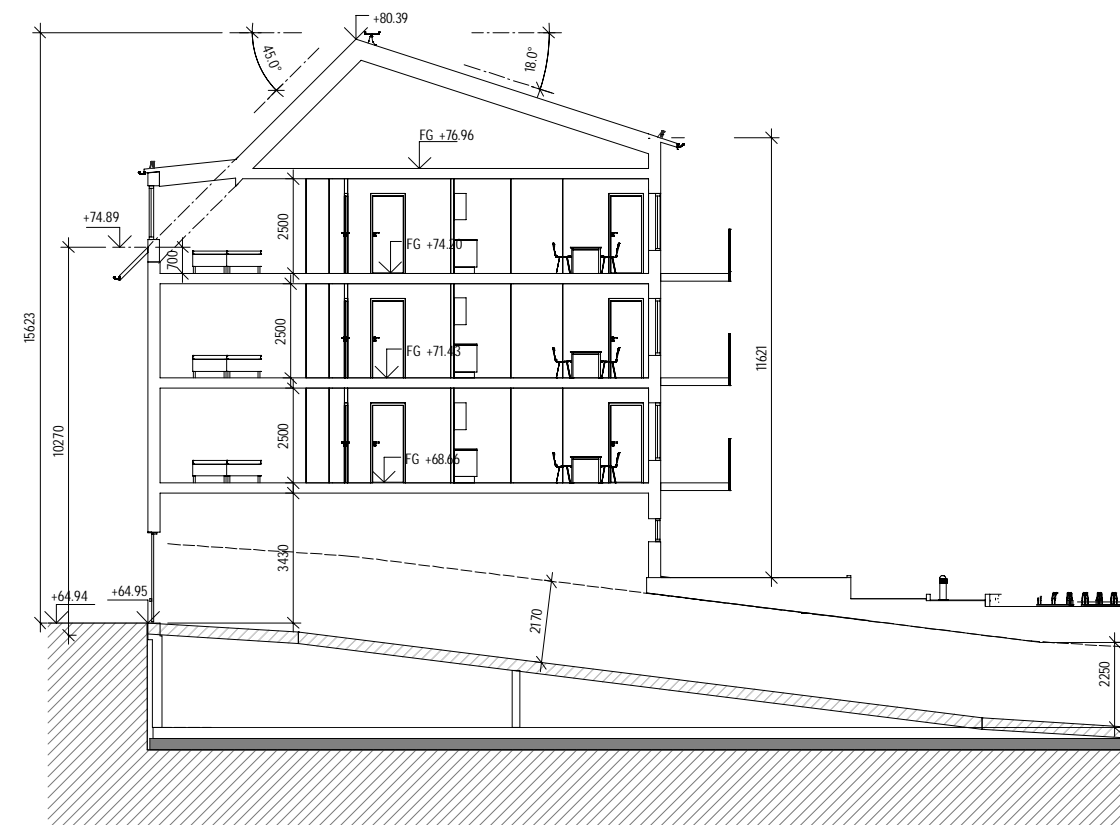
SEKTION F-F BL 1 : 100
