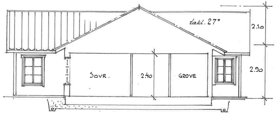
SEKTION SK. 1:100
