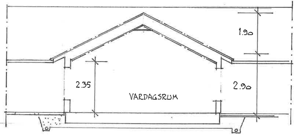
SEKTION SK. 1:100
