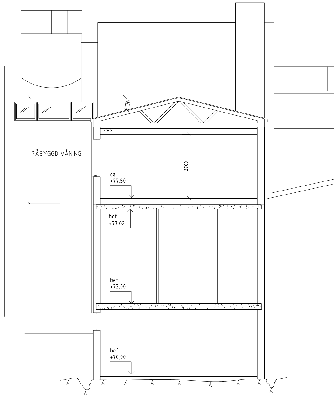
SEKTION A-A
