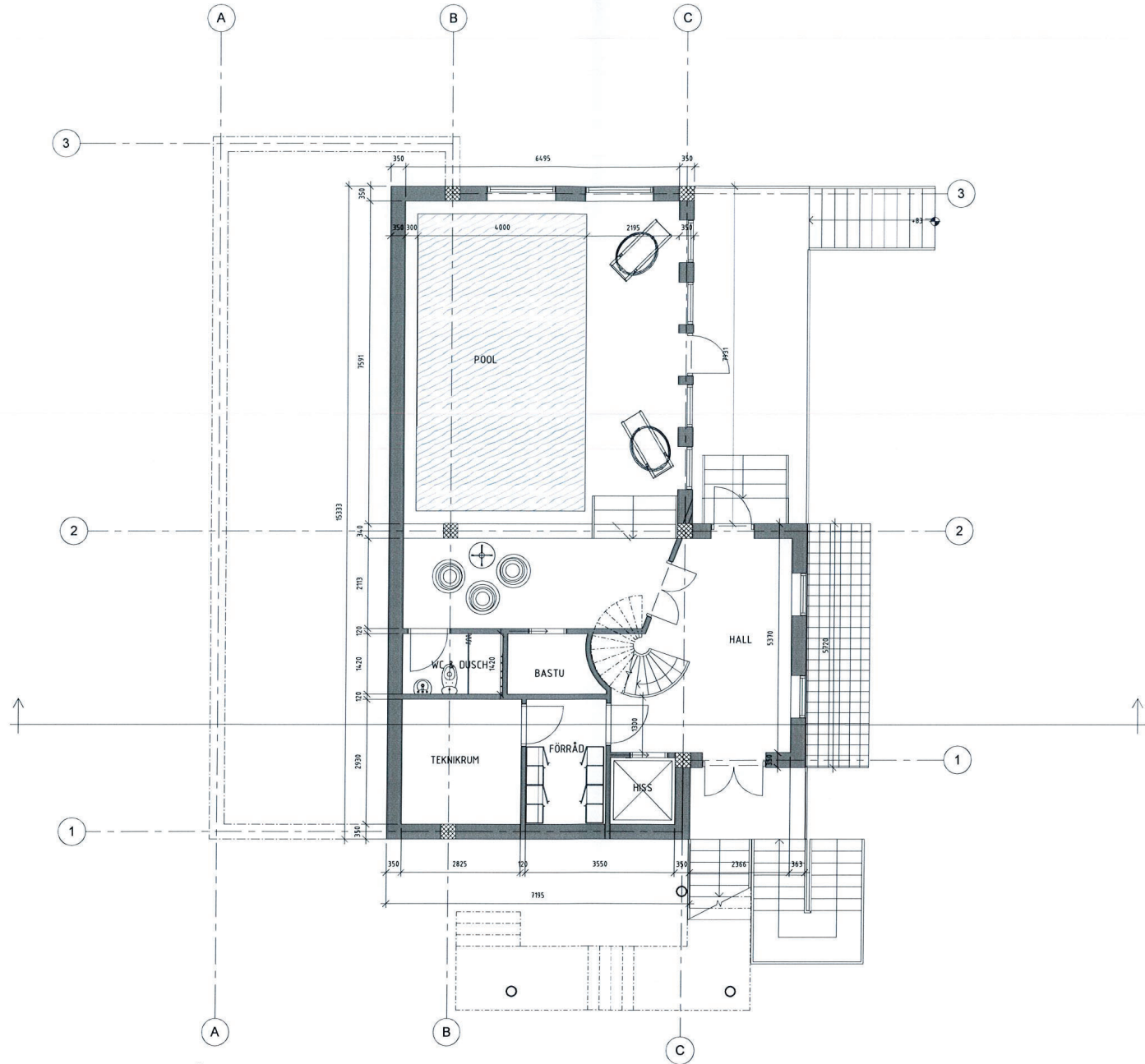
1 SOUTERRÅNG 1 : 50
