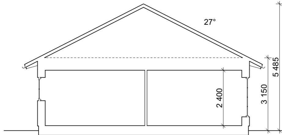
Sektion A-A 1:100
