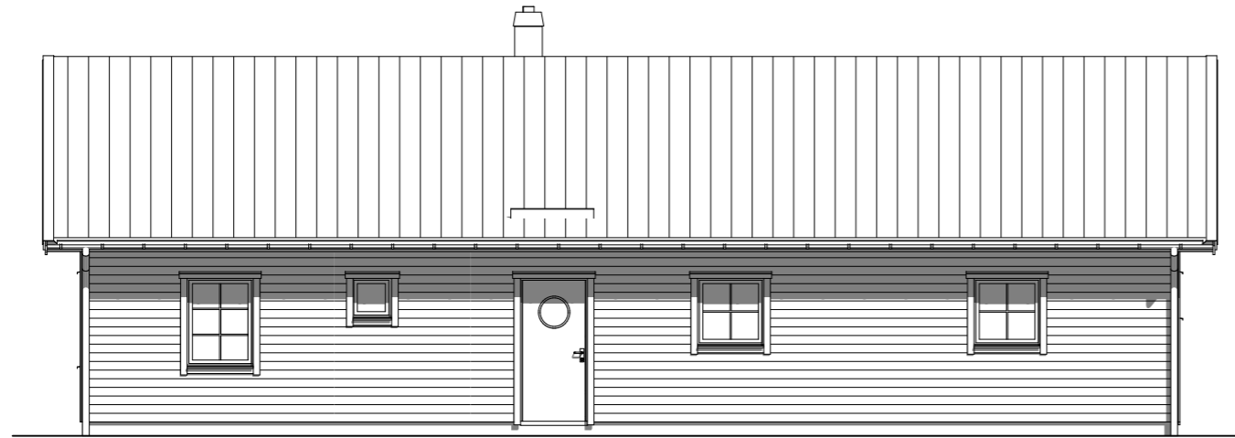
Fasad F1 1:100
