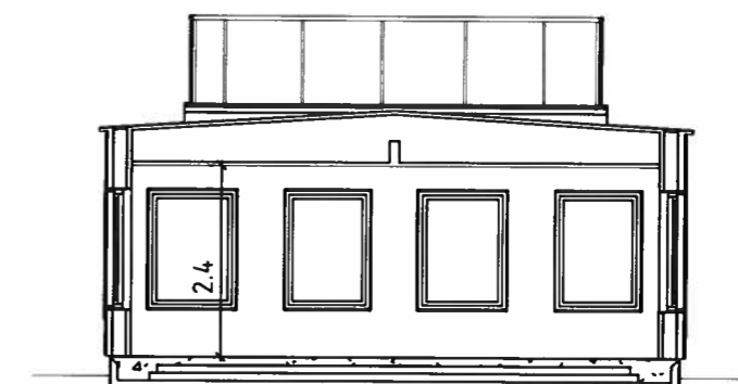
SEKTION C - C
