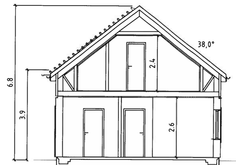
SEKTION B - B
