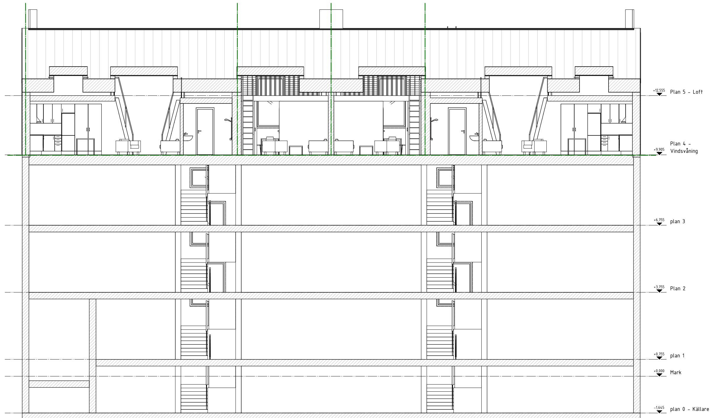
LÄNGDSEKTION B-B
