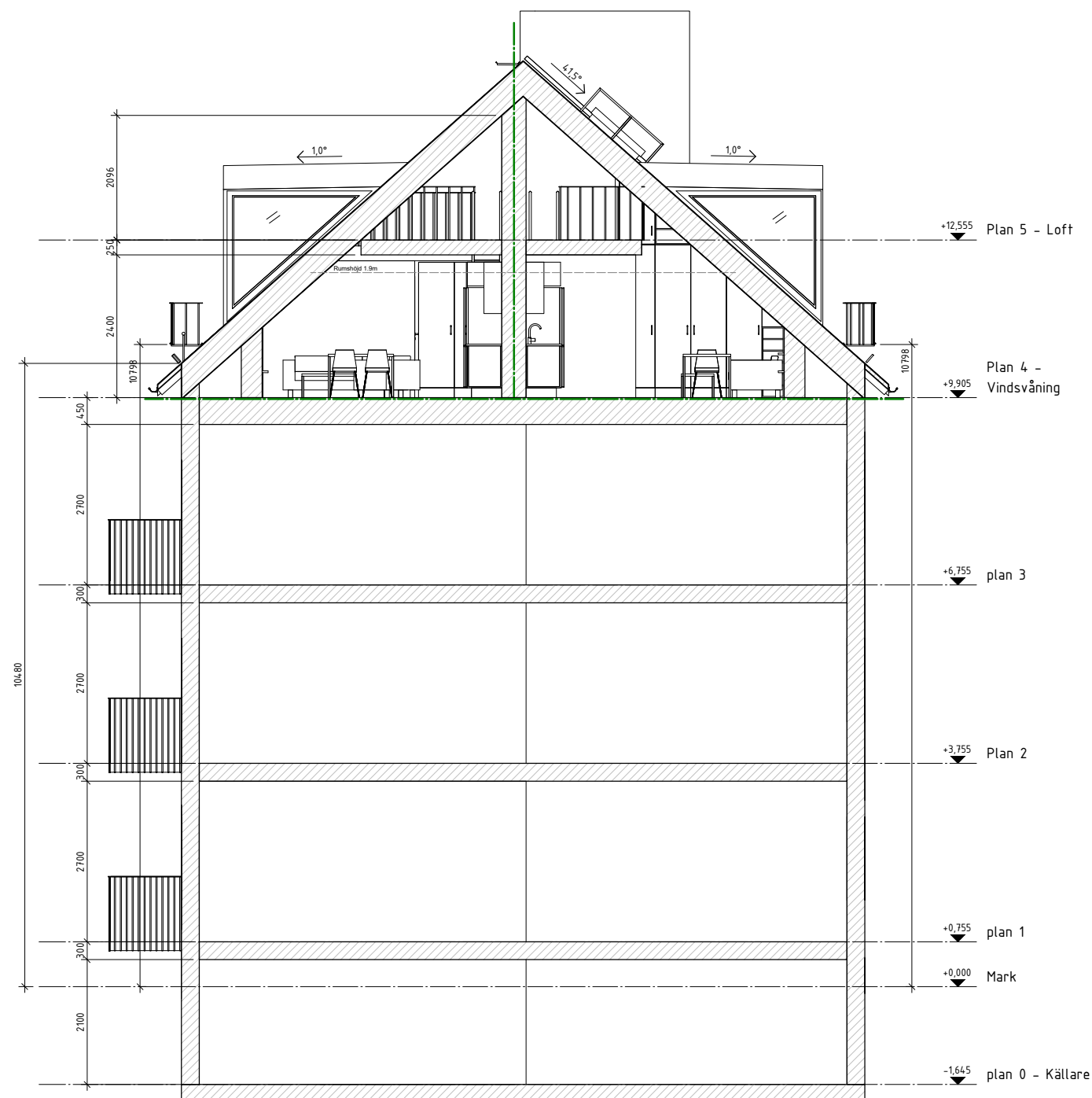
TVÄRSEKTION A2-A2
