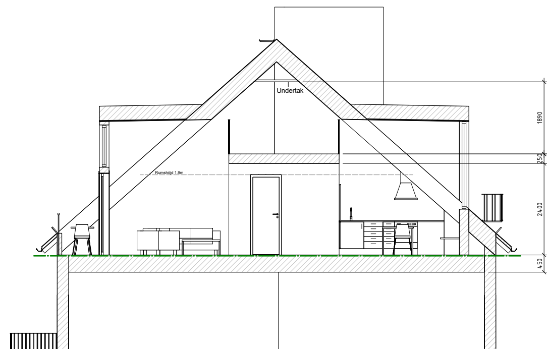
TVÄRSEKTION A1-A1
