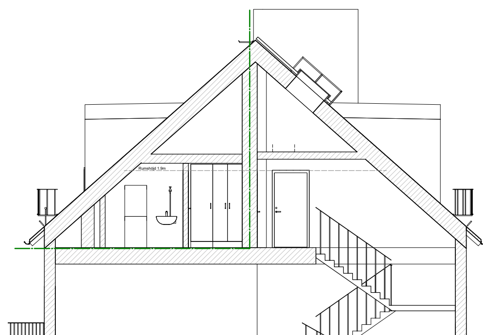
TVÄRSEKTION A3-A3
