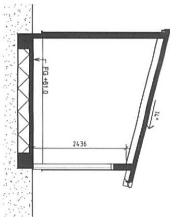
SEKTION A
