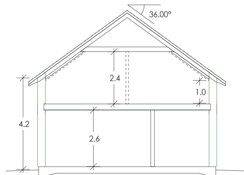
Sektion A-A
