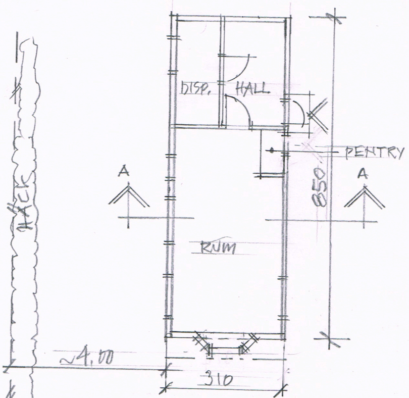
PLAN BR 26,3 m 2
