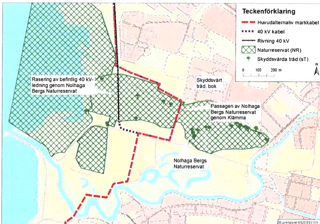
Figur 2. Huvudalternativ för planerad 132 kV-ledning och kablifiering av befintlig 40 kV-ledning genom Nolhaga Bergs naturreservat, samt rasering av befintlig 40 kV-ledning genom Nolhaga Bergs naturreservat.
