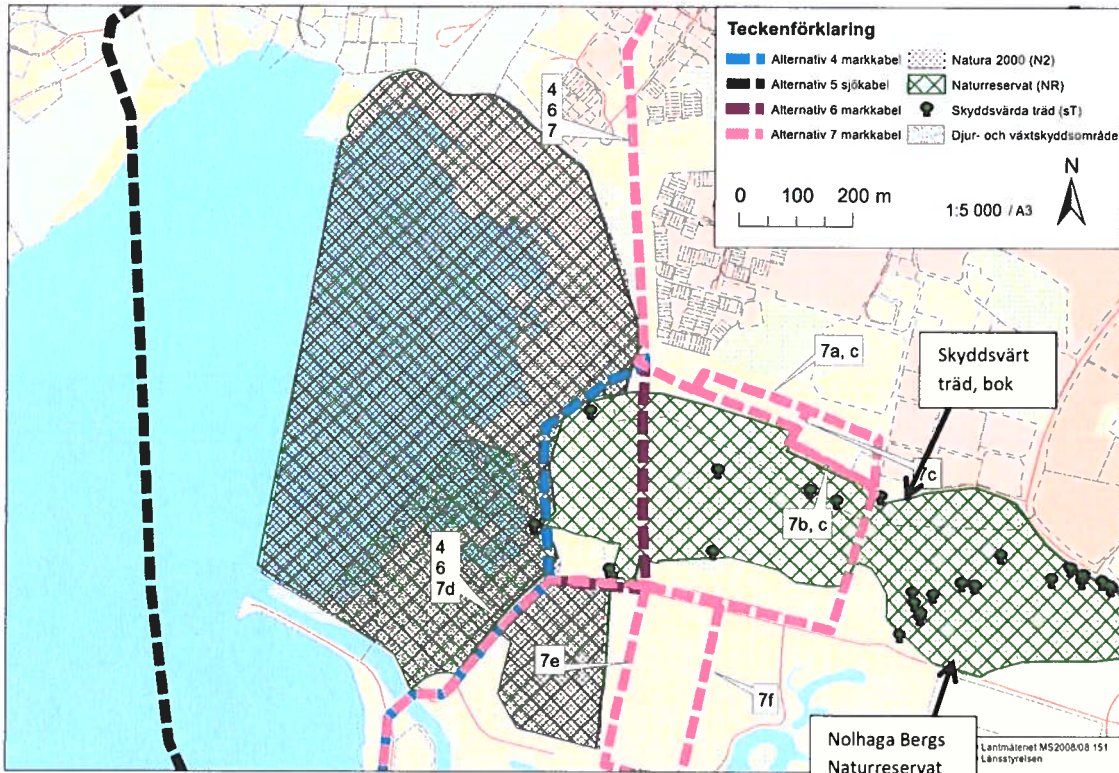
Figur 1. Översikt alternativa ledningsträckningar för planerad 132 kV-ledning genom Nolhaga bergs naturreservat.
