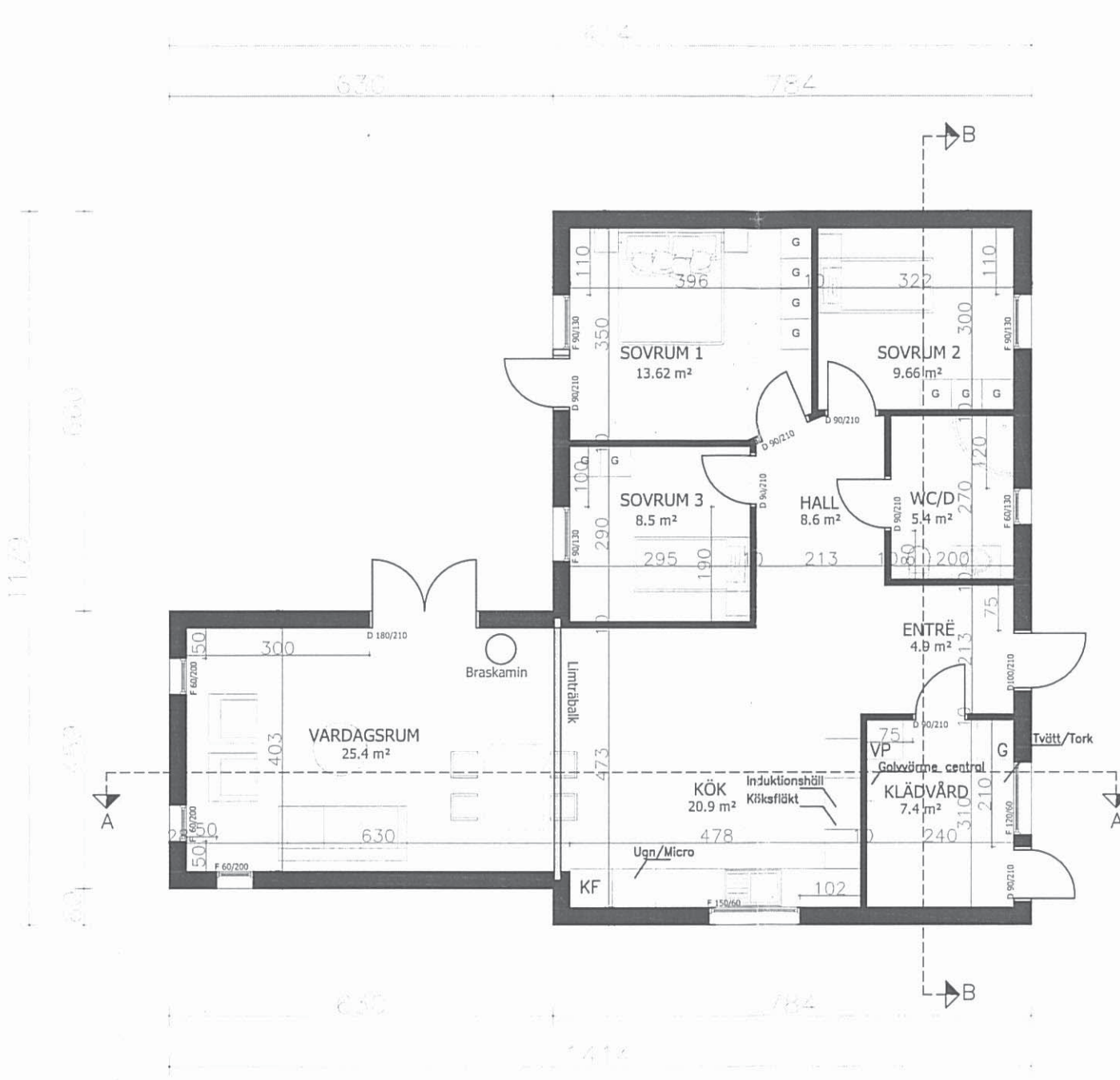
ENTRÉPLAN BOA 107.04 m 2 BYA - Byggnadsarea 119.86 m 2
