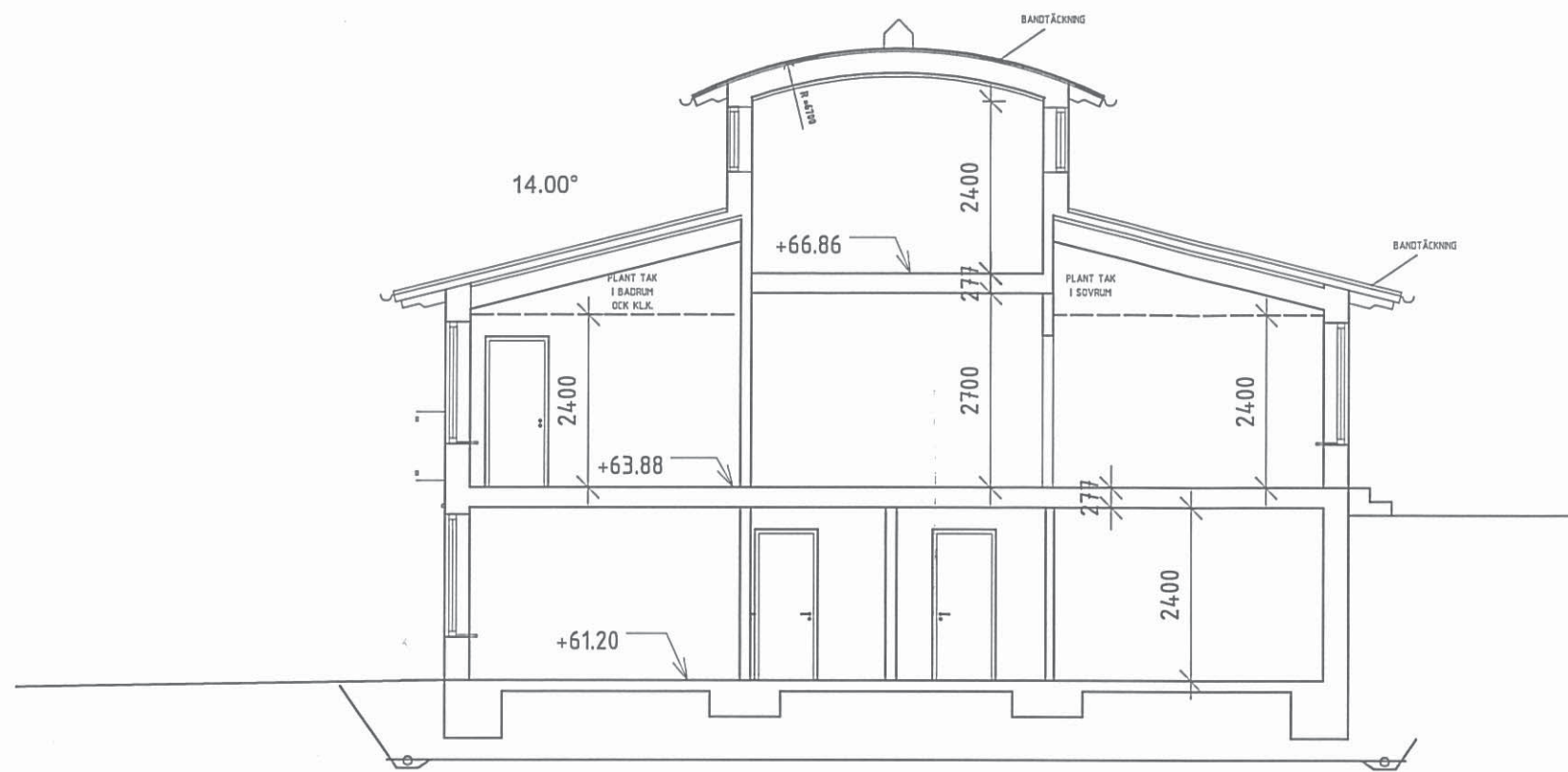
SEKTION 1
