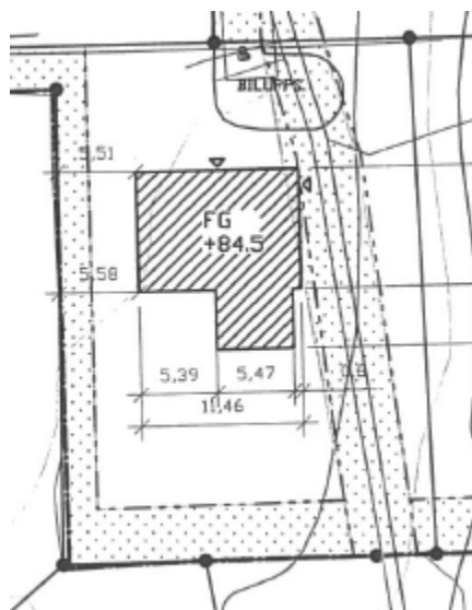
Nybyggnadskarta för bygglovet
