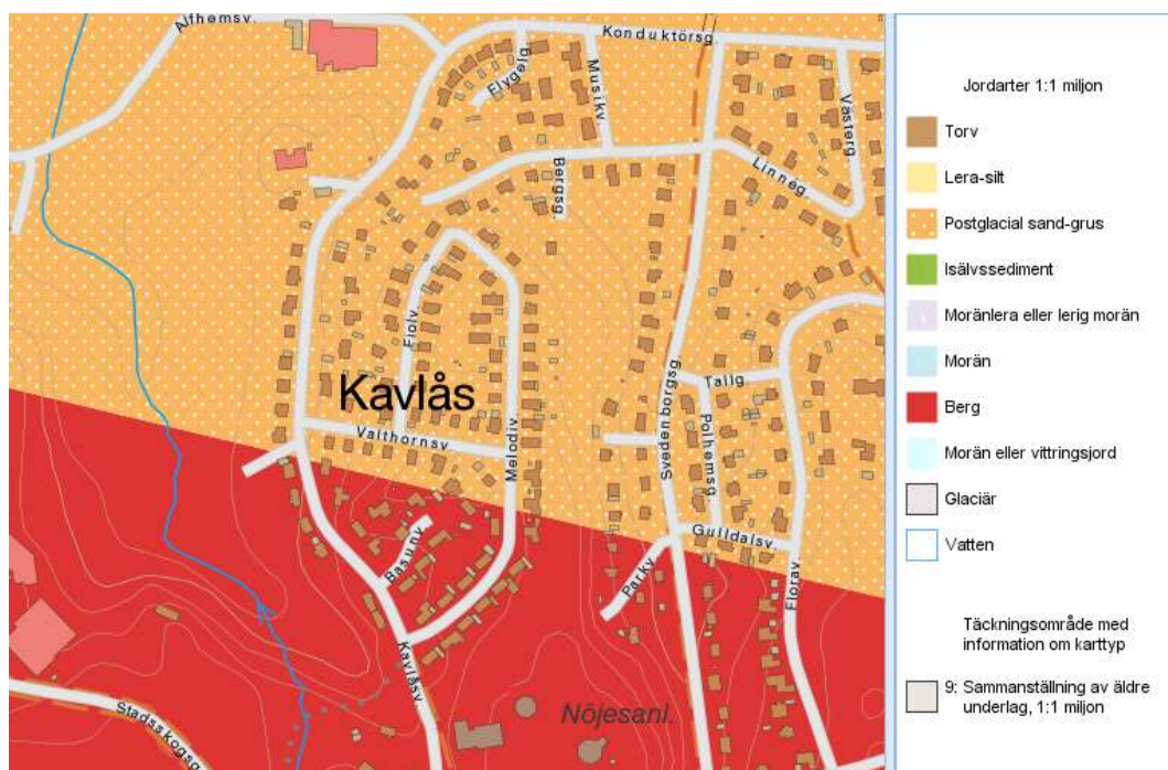
Bild 1. SGU:s jordartskarta.
