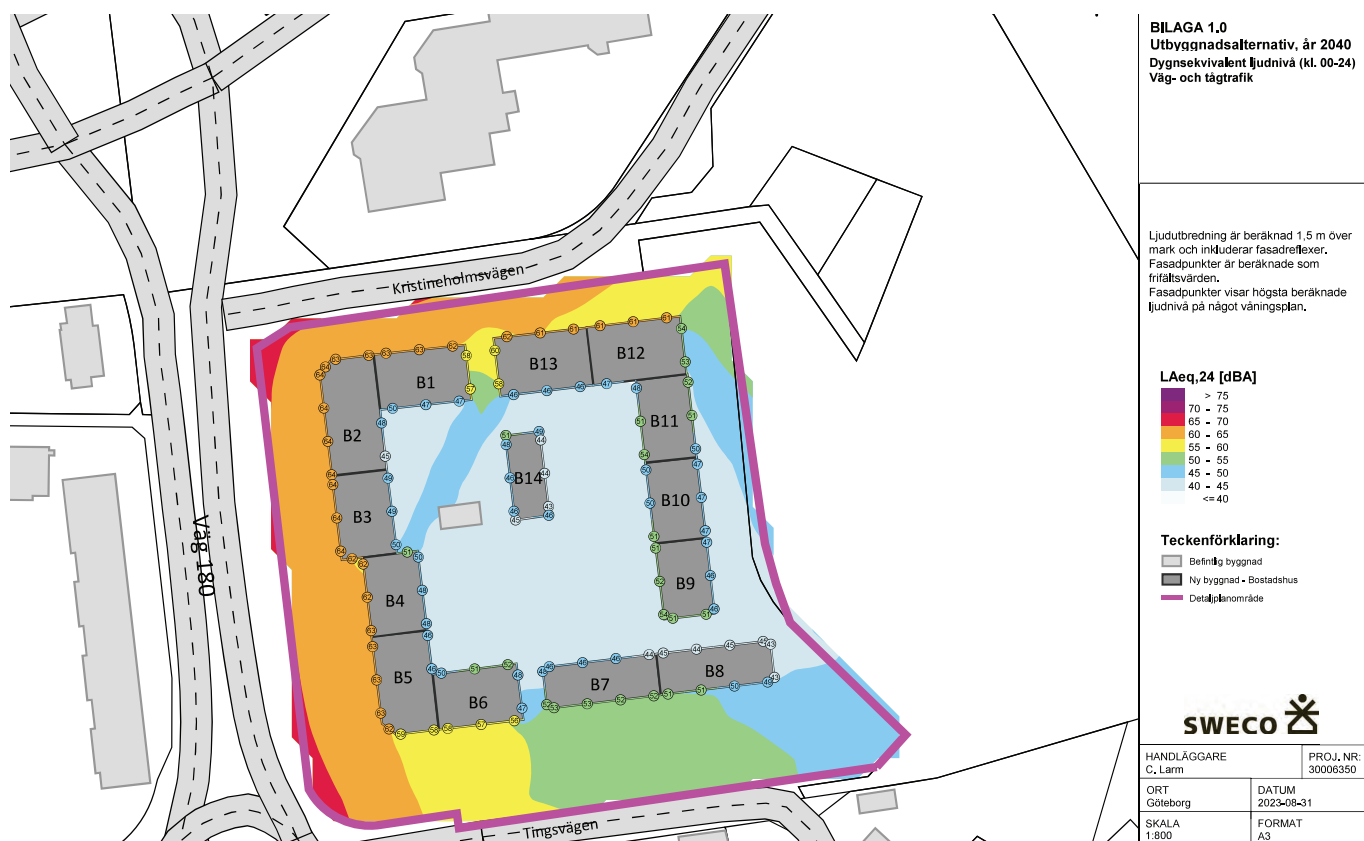
Figur 31 - Trafikbullerberäkning som visar dygnsekvivalent ljudnivå för väg- och tågtrafik år 2040 (Sweco, 2023-01-19)
