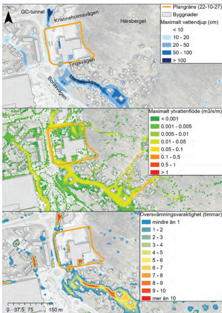
Figur 28 - Maximalt vattendjup och ytvattenflöde samt varaktighet på översvämning vid ett modellerat 100-årsregn med klimatfaktor 1,35 (Sweco, 2022-04-21), figur från dagvatten- och skyfallsutredning (Sweco, 2023-08-31).
