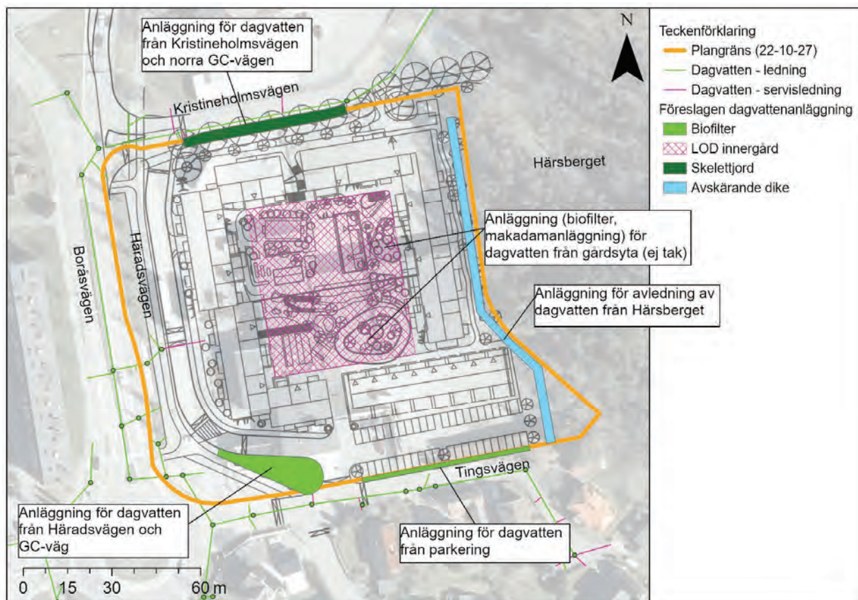
Figur 29 - Schematisk bild av föreslagen dagvattenhantering inom planområdet (Sweco, 2023-01-19).
