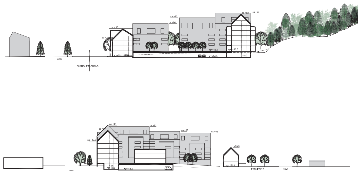
Figur 10 - Sektioner som visar hur föreslagen bebyggelse förhåller sig till omgivande bebyggelse samt berget i öster. Sektioner från gestaltningsprogrammet (Krook&Tjäder, 2023-08-31).
