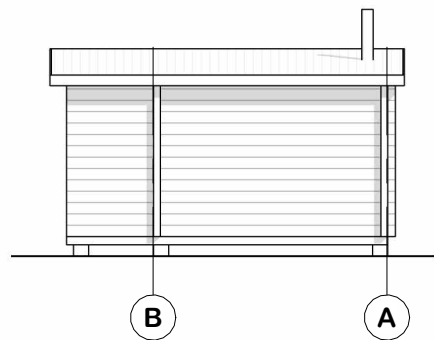
1 SÖDER 1 : 100
