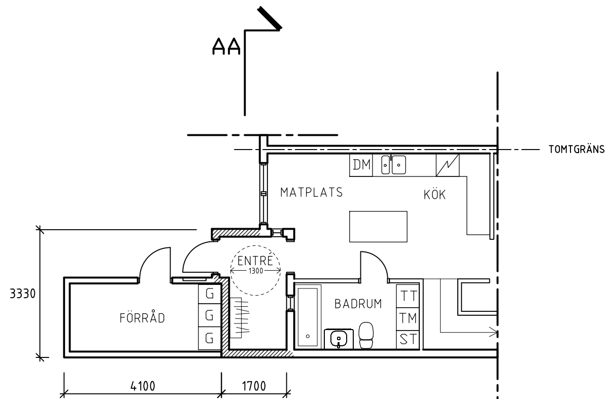
PLAN 1 1:100
