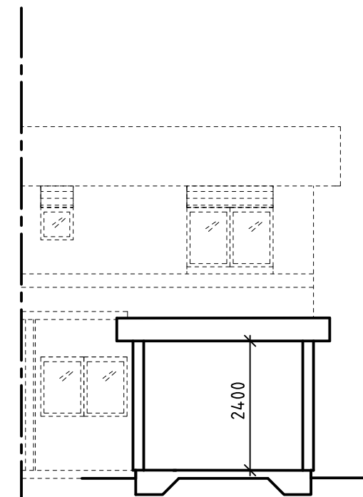
SEKTION AA 1:100
