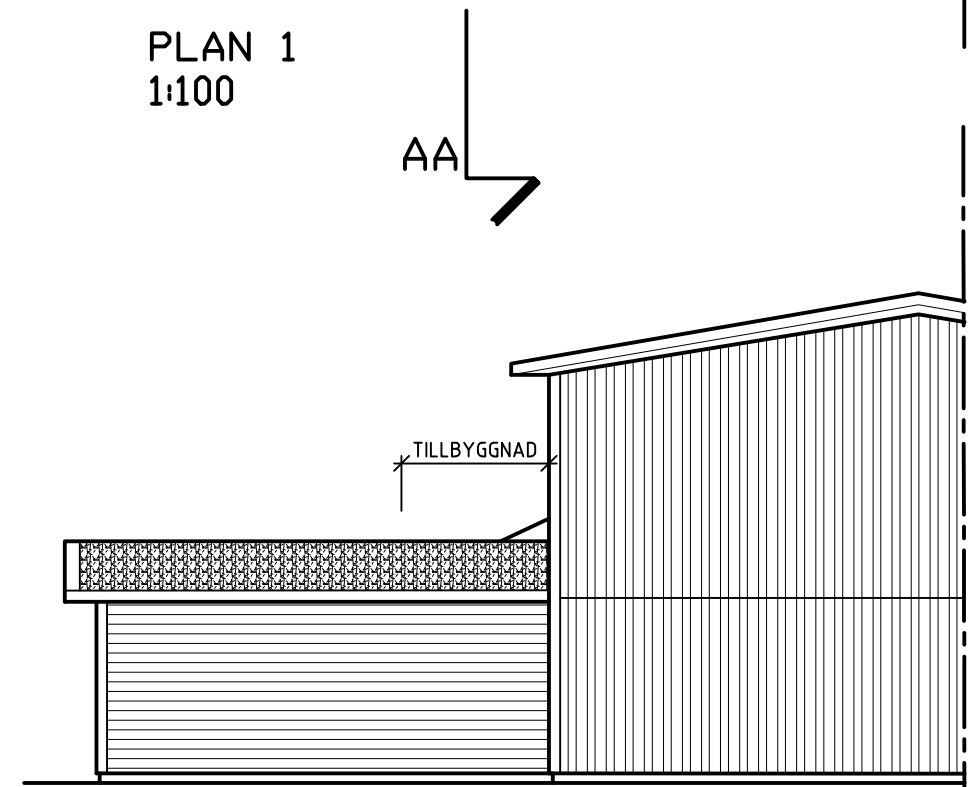
FASADRITNING MOT SÖDER 1:100
