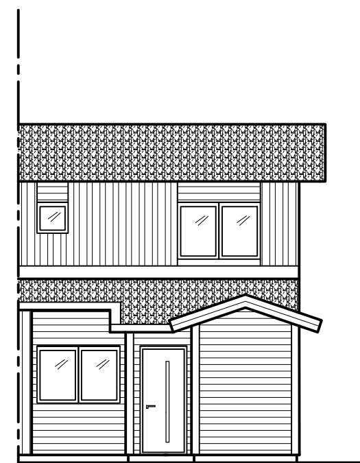
FASADRITNING MOT VÄSTER 1:100
