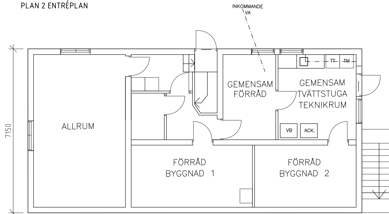
PLAN 2 ENTRÉPLAN
