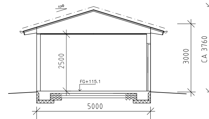
SEKTION
