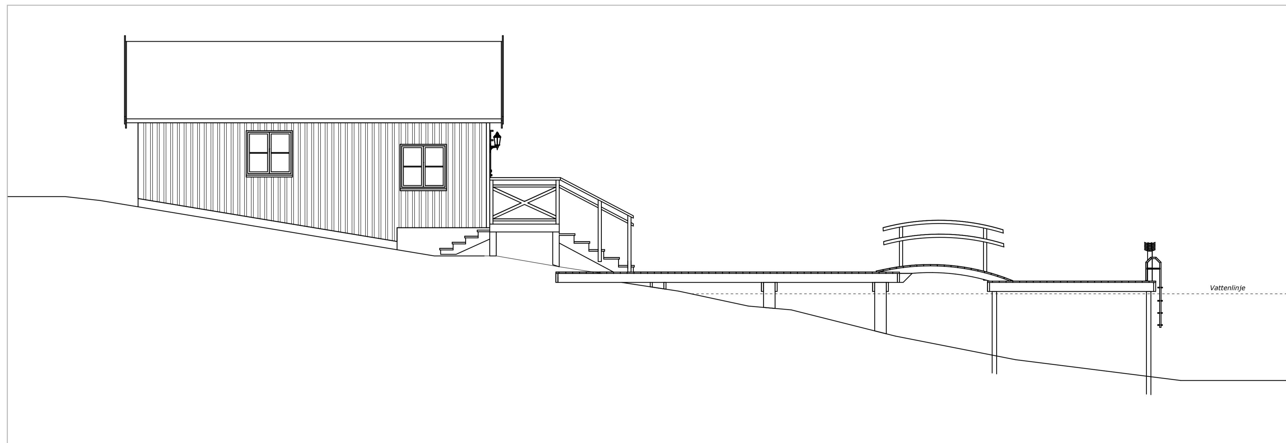
Elevation Öst
