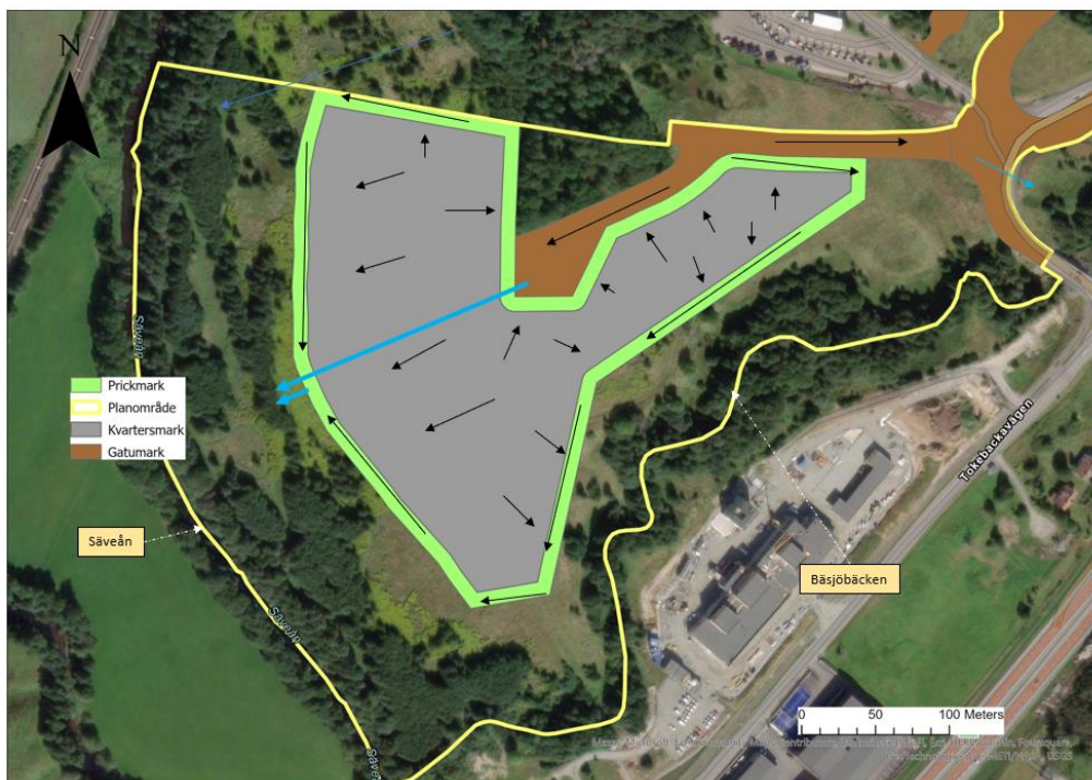
Figur 27. Delområdet i söder. Riktning på avrinningsvägar är enligt svarta pilar. Renat dagvatten från allmän platsmark och kvartermark (blåa pilar) mynnar ut i Säveån. Delar av vägen som vetter österut avrinner mot Bäsjöbäcken. Avrinning från naturmarken uppströms bör ledas förbi planområdet.
