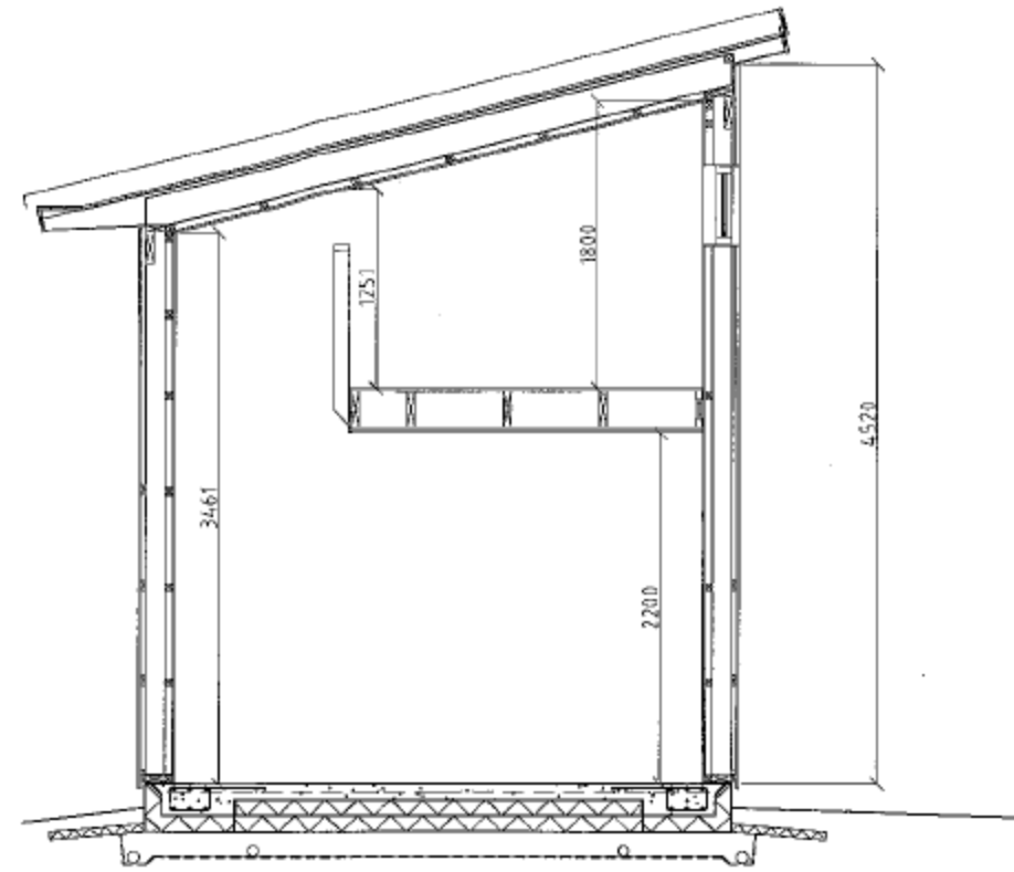
Sektion A-A
