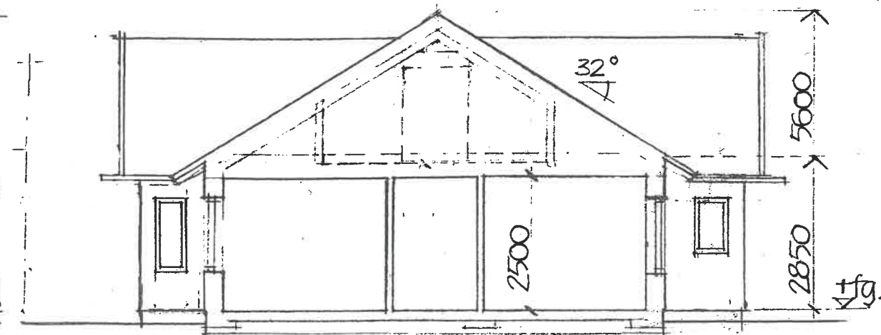
sektion A
